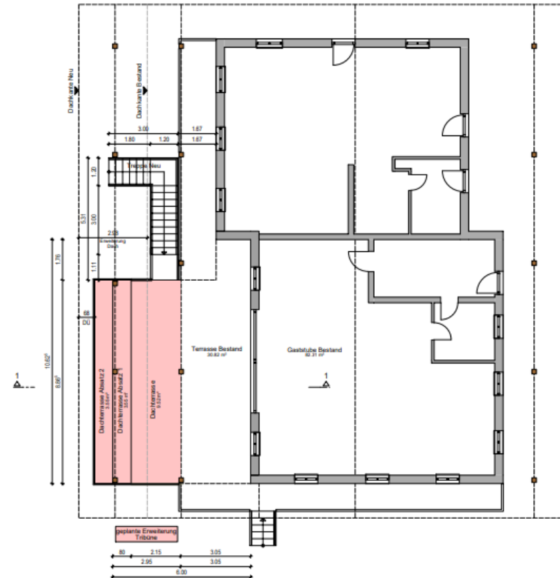
Grundriss - Erdgeschoss 1:100
