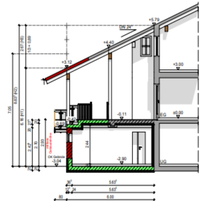
Schnitt 1-1 1:100
