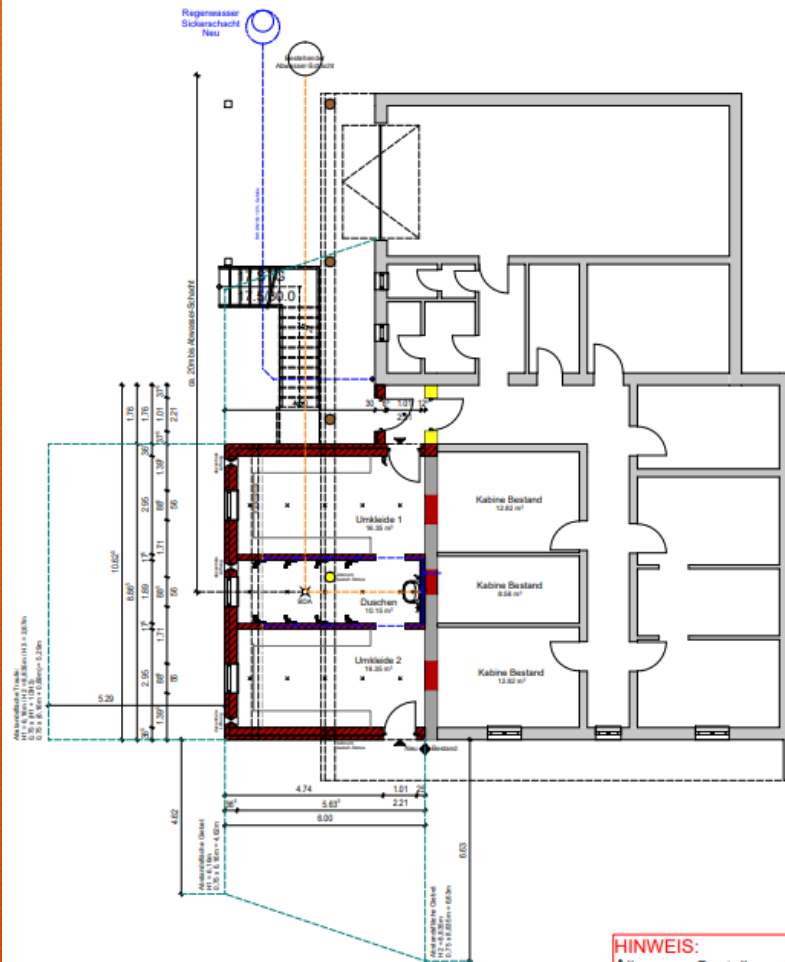
Grundriss - Untergeschoss 1:100
